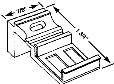
AWV 53 SUPERIOR CLIP
