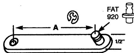
JALOUSIE LINK W/E-RING STUD
