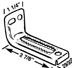
CDF 29 JAMB BRACKET
