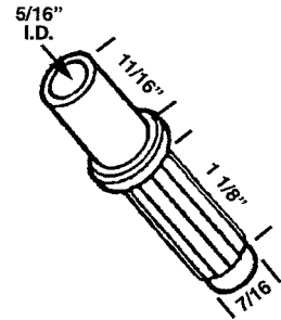
CDF 130 TOP PIVOT GUIDE
