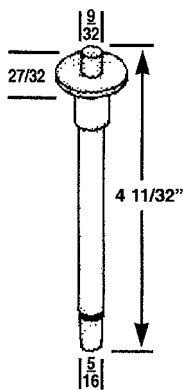
CDF 624 FENESTRA GUIDE
