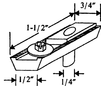
CDF 711 BOTTOM PIVOT BLOCK
