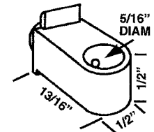
CDF 718 ROD CLAMP
