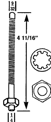
CDF 630 NATIONAL BOTTOM PIVOT
