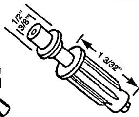
CDF 111 GUIDE PIN
