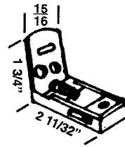
CDF 51 JAMB BRACKET
