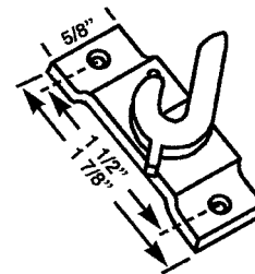
CDF 47 SHUTTER DOOR BRACKET
