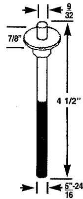
CDF 625 FENESTRA BOTTOM PIVOT
