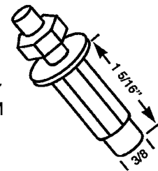
CDF 137 BOTTOM PIVOT
