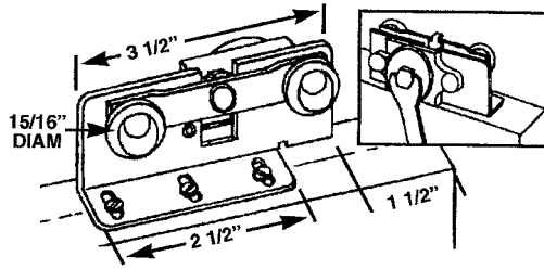
CDB 191 DOUBLE ROLLER POCKET DOOR
