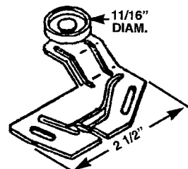
CDB 102 BACK HANGER
