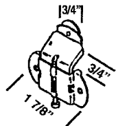
CDB 66 CLOSET DOOR HANGER BACK
