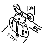
CDB 67 CLOSET DOOR HANGER FRONT
