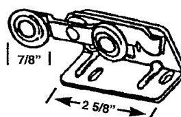
CDB 53 DOUBLE ROLLER
