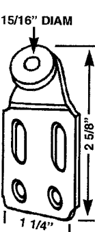
CDB 146 HANGER
