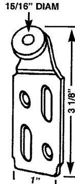
CDB 138 HANGER
