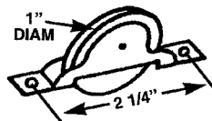
CDB 61 CLOSET ROLLER
