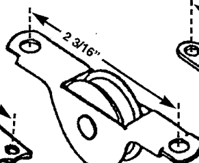
CDB 122 SHEAVE
