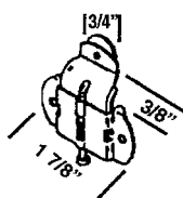
CDB 63 CLOSET DOOR HANGER FRONT
