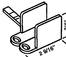
CDB 193 POCKET DOOR GUIDE ADJ. TO 1 3/4\"/>
