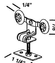
CDB 44 DOUBLE ROLLER
