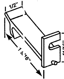
SWP 28 ALENCO BOTTOM GUIDE
