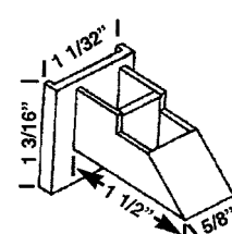
HWP 847 TOP GUIDE
