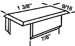
HWP 790 APL END CAP
