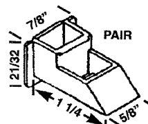
HWP 143 NUAIRE TOP GUIDE
