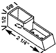
HWP 95 TOP GUIDE
