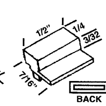
BACK HWP 217 VENT GUIDE
