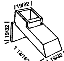
HWP 793 HOWARD TOP GUIDE
