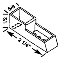
HWP 94 TOP GUIDE
