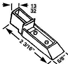
HWP 879 TOP GUIDE
