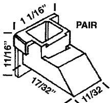
HWP 142 NUAIRE GUIDE
