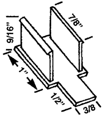
HWP 862 ROLLYSON GUIDE
