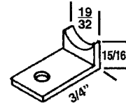
HWP100 GUIDE
