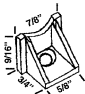
HWP 215 GUIDE
