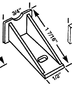
HWP 832 GUIDE
