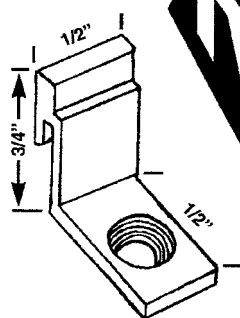
HWP 296 GUIDE
