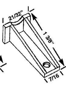
HWP 333 GUIDE
