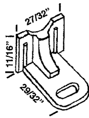
HWP 370 GUIDE
