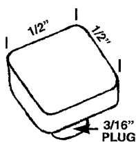
HWP 257 GUIDE
