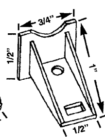
HWP 321 WALLACE GUIDE
