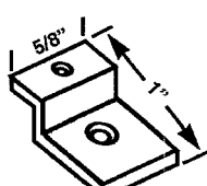
HWP 928 GUIDE
