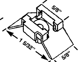
HWP 369 GUIDE
