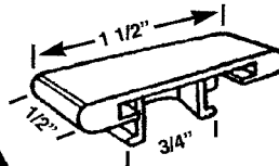
HWP 703 GUIDE
