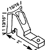
HWP 135 FOOT
