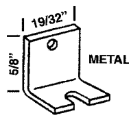
HWP 881 ANGLE CLIP
