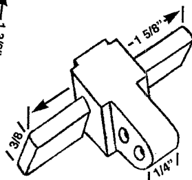
HWP 303 PIVOT BAR
