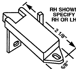
RH SHOWN SPECIFY RH OR LH HWP 803 ACORN PIVOT LATCH
