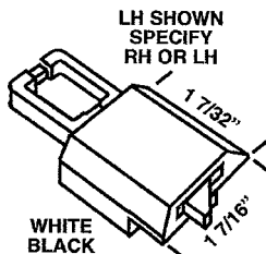
LH SHOWN SPECIFY RH OR LH HWP 700 KELLER SLIDE LATCH TILT WINDOW
