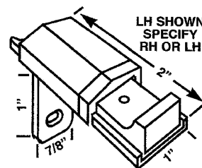
LH SHOWN SPECIFY RH OR LH HWP 789 TILT LATCH
