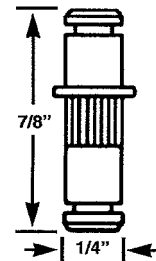
FAS 51 GENERAL LONG STUD
