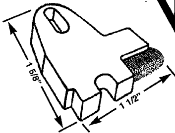
PDG 77 PATIO DOOR GUIDE
