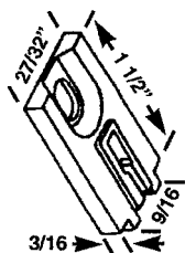
PDG 3 DARYL TOP GUIDE
