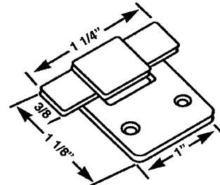
PDG 84 BELLEVIEW DOOR GUIDE
