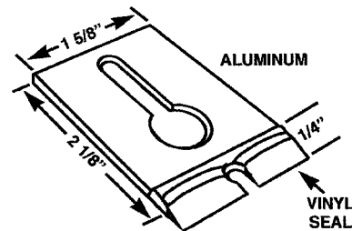
PDG 85 KELLER BOTTOM SWEEP
