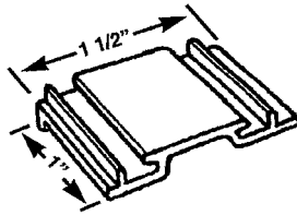
PDG 80 HAR CAR TOP GUIDE
