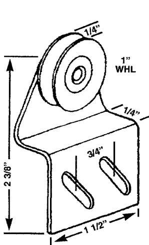
PSR 37 STEEL BB ROLLER ASMB
