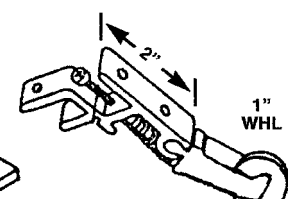
PSR 20 EXTR CORNER ASMB
