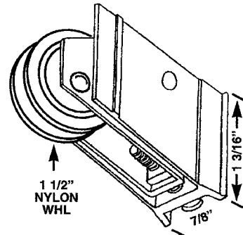
PSR 62 ROLLER ASMB
