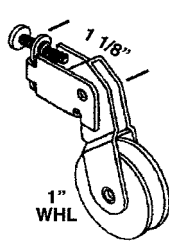
PSR 86 PEACHTREE ASMB
