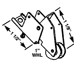
PSR 80 ROLLER ASMB
