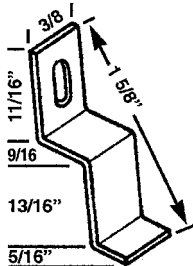
WSC 197 VT PGT CLIP
